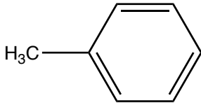
Toluol
