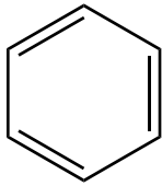
Benzol
