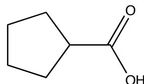
Carbonsäure Cyclopentancarbonsäure
