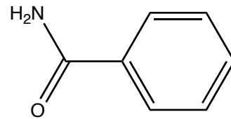
Benzamid
