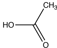
Essigsäure
