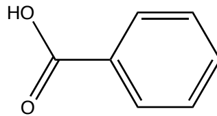
Benzoessäure
