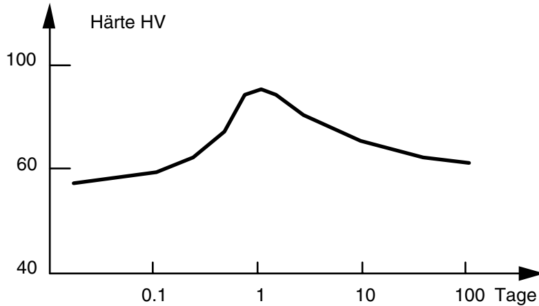
Fig.: Warmaushärtung von AlCu4 bei 190°C
