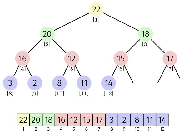
Abbildung 4.1: Algorithmus Aufsteigen
