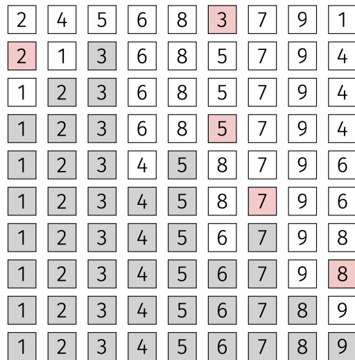
Abbildung 5.5: Quicksort
