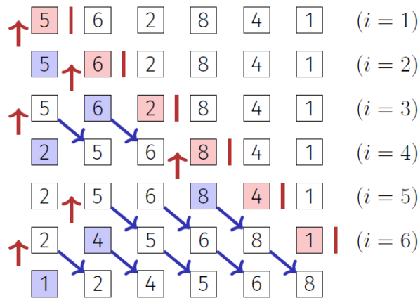
Abbildung 5.3: Insertionsort
