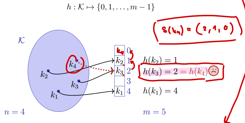
Abbildung 4.3: Schlüsselmengebildung auf Hashtabellenindizes
