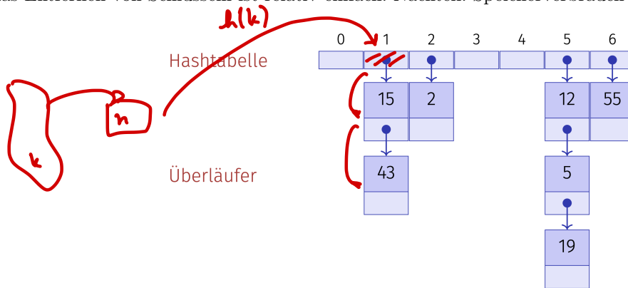
Abbildung 4.2: Hashing mit Kollision h(k_3) = h(k_4)
