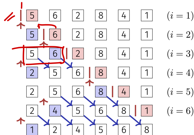
Abbildung 5.3: Insertionsort
